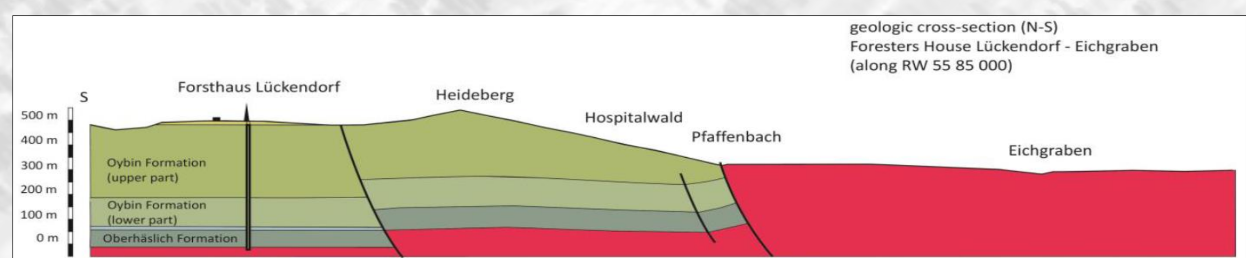
Abb. 3: Geologischer Schnitt durch Lausitzer Überschiebung in Höhe Lückendorf (Quelle: Thomas Voigt; Universität Jena)
