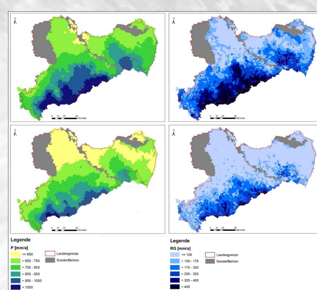
Abb. 4: Langjähriger mittlerer Niederschlag (links) und Grundwasserkomponente (rechts) für 1961-1990 (oben) und 2071-2100 (unten) der Realisierung 99 A1B, WETTREG2010 (LfULG Schriftenreihe 08/2016)
