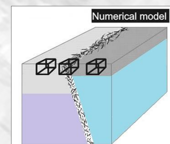
Abb. 5: Diskretisierung Numerisches Modell (verändert nach Bense et al. 2013)
