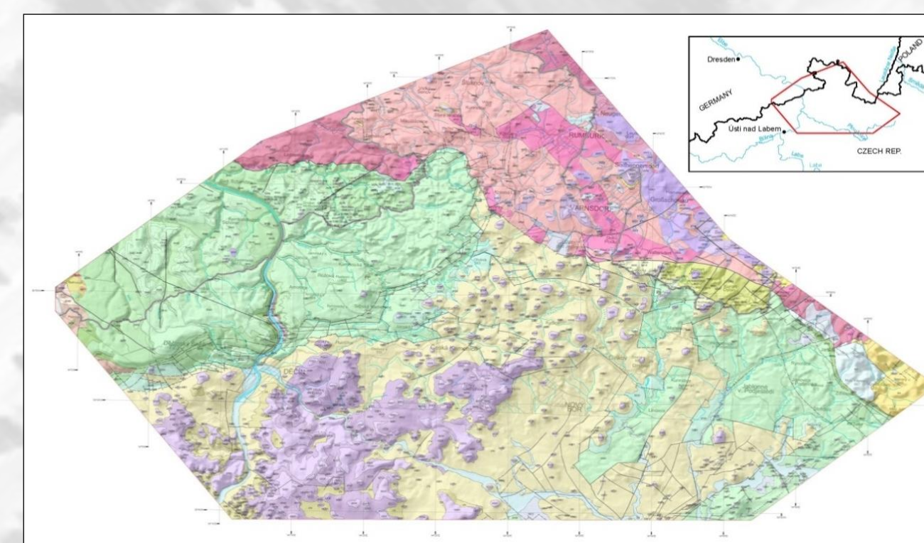
Abb. 6: 2D-Geologische Karte des Untersuchungsgebietes
