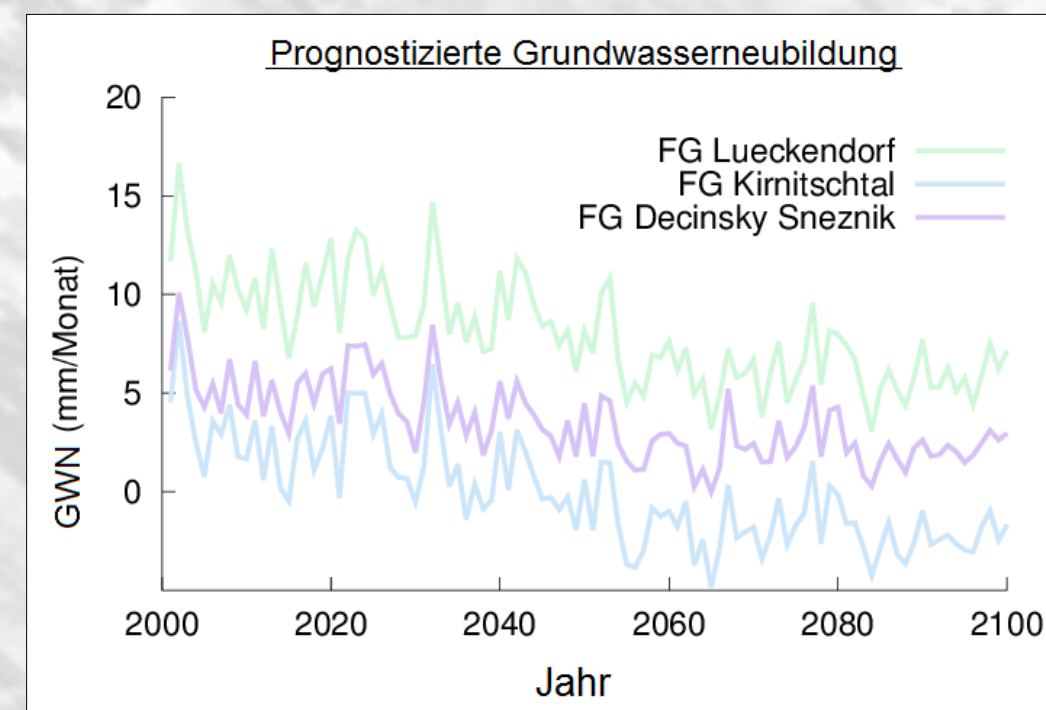
Abb. 1: Gleitendes 12-Monatsmittel der Grundwasserneubildung auf Einzugsgebietsebene (Median des WEREX-V-Ensembles aus dem Projekt KLiWES)
