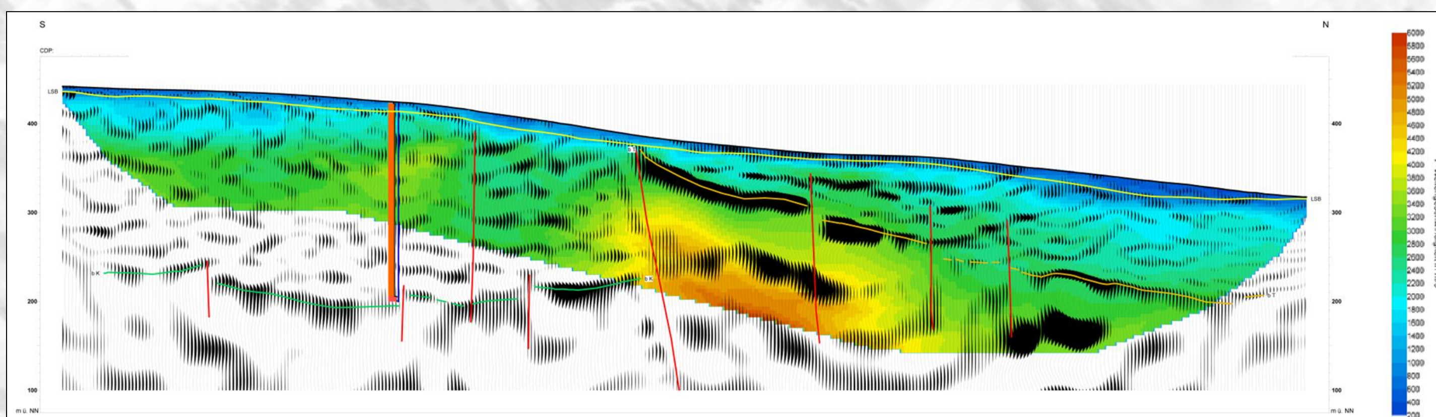
Abb. 7: Seismisches Profil zwischen Hartau und Lückendorf (Zittauer Gebirge)
